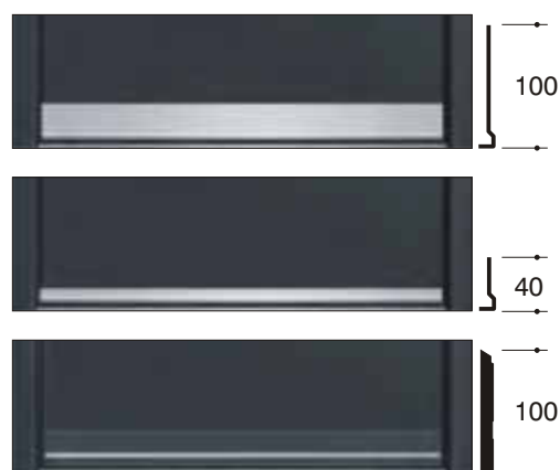
Wetterschenkelprofil - Edelstahl matt
