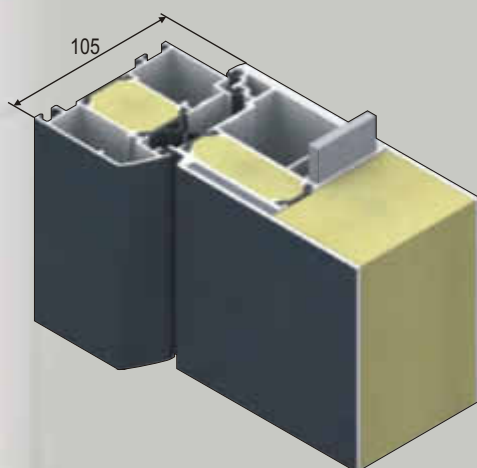
AT 100 STANDARD FORM MIT VERSTÄRKUNG
