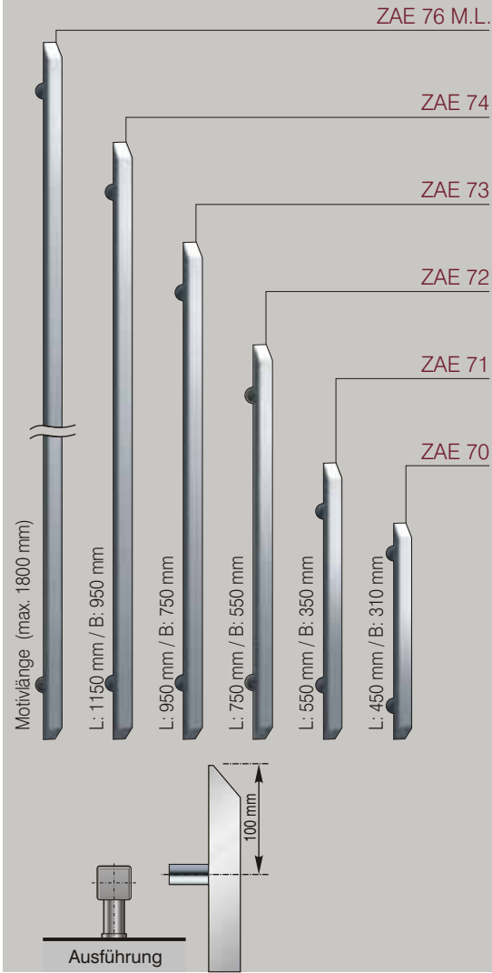
Stossgriff aussen - Serie Quadra - Edelstahl matt
