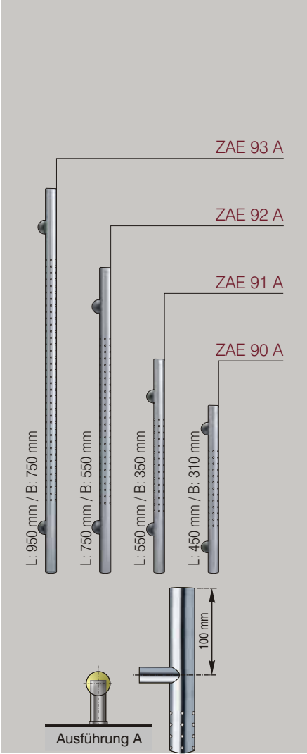
Stossgriff aussen - Serie Punkt - Edelstahl matt
